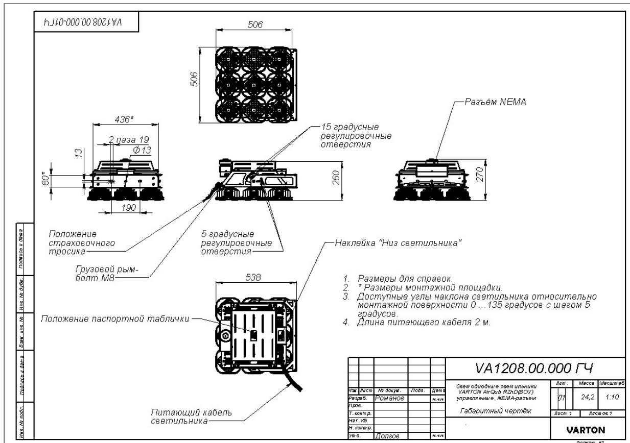
Габаритный чертёж светильников VA1208.00.000 AirQub RZhD 660 Вт
